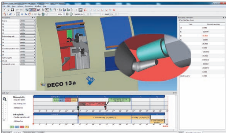
Mastercam Swiss Expert идеально подходит для изготовления медицинских изделий – в частности абатментов. Простота программирования и большой набор функциональных возможностей позволяют производить обработку таких сложных и ответственных деталей
